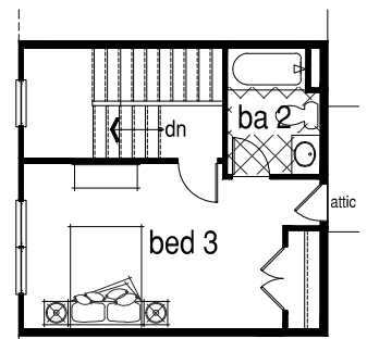
Optional Bed 3 / Bath 2
